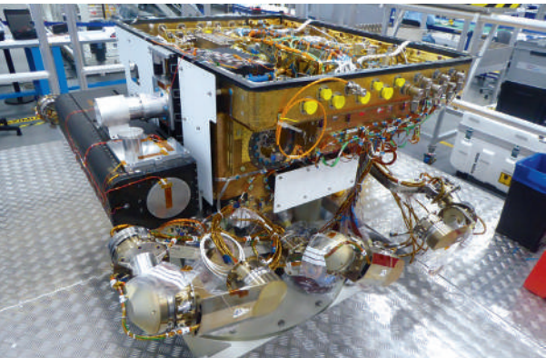
Radiadores y sistema de transmisión térmica instalados en el STM de ExoMars
