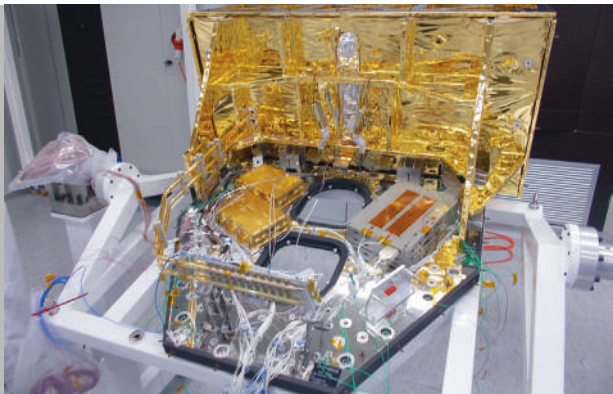
Subsistema criogénico del instrumento 3MI de la misión MetOP SG
