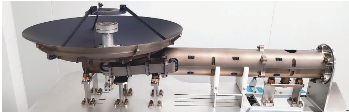
Sistema completo de la antena de media ganancia de JUICE_©SENER
