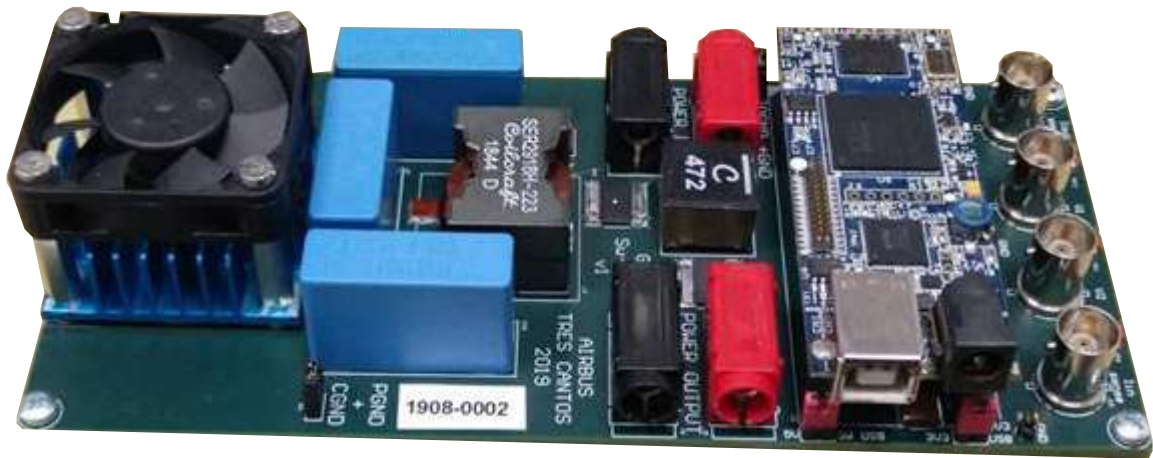
Modelo para tests dinámicos del convertidor a base GaN
