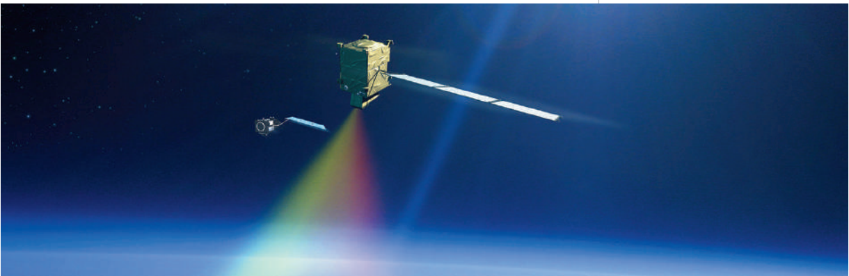
FLEX proporcionará mapas globales de fluorescencia (© ESA/ATG medialab)
