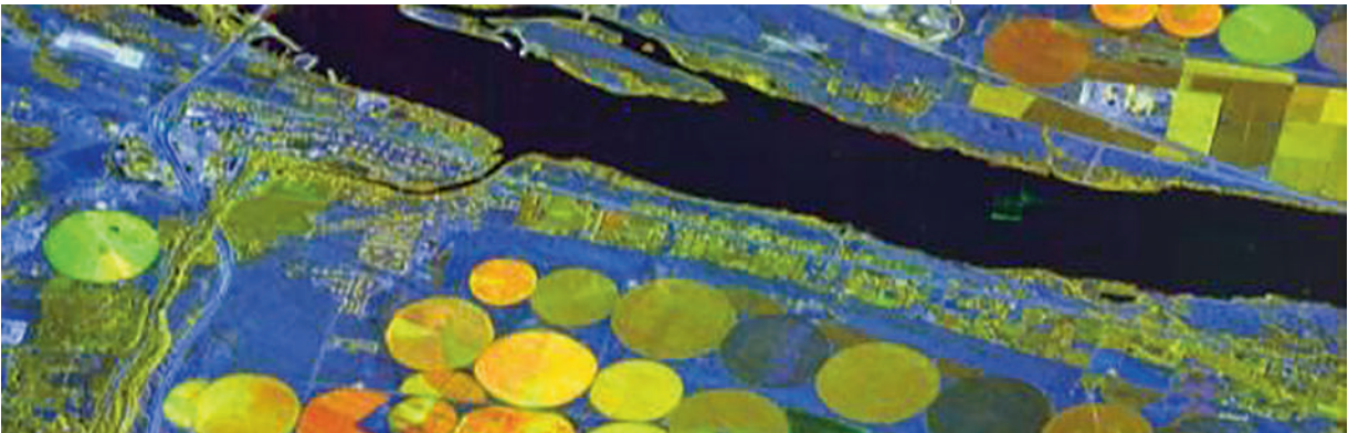
Aplicación de datos satelitales para la monitorización de cultivos
