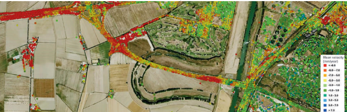
Estudio de deformaciones del terreno mediante tecnología SAR
